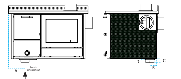
Dimensions en mm - Thermo-cuisinière à bois avec sortie fumées à droite
