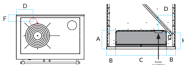
Dimensions en mm - Cuisinière à bois avec sortie fumées à droite
