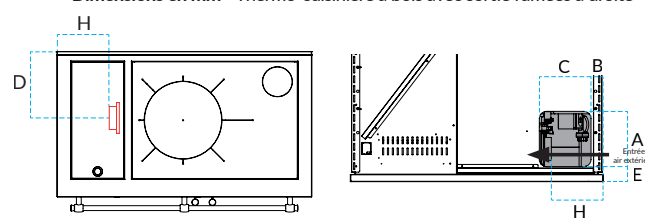
Dimensions en mm - Thermo-cuisinière à bois avec sortie fumées à droite
