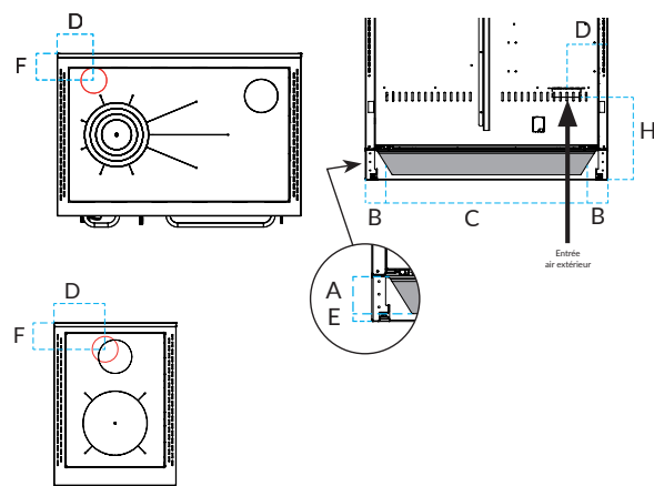
Dimensions en mm - Cuisinière à bois avec sortie fumées à droite
